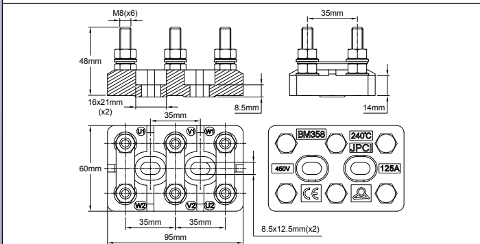
Модель 125 А 450 В (расстояние между клеммными зажимами 35 мм, винты М8)
