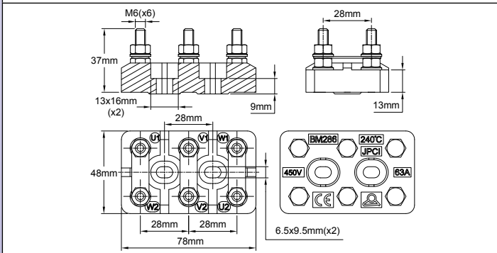
Модель 63 А 450 В (расстояние между клеммными зажимами 28 мм, винты М6)
