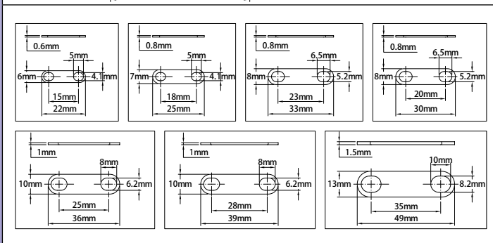
Навесные перемычки из латуни для клеммных колодок электродвигателя
