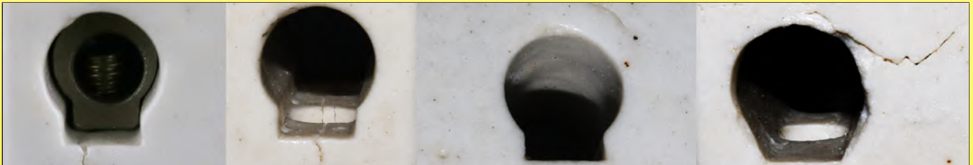
Примеры трещин на фарфоре C111
