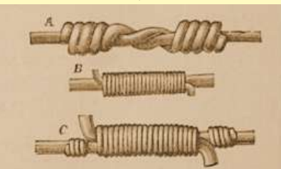
Соединение электрических проводов путем сплетения в 1892 г. (Manuel pratique de l'installation de la lumière électrique. Installés privées, J.-P. Anney)
