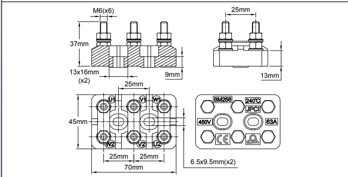
Модель 63 А 450 В (расстояние между клеммными зажимами 25 мм, винты М6)
