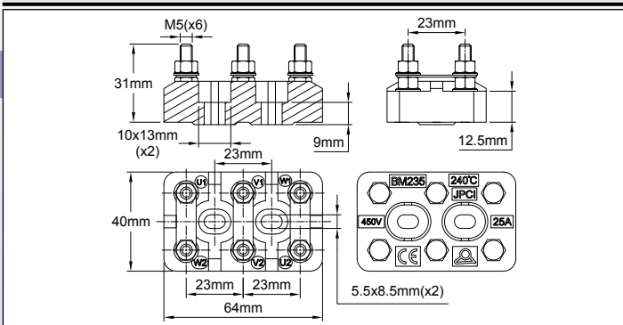
Модель 25 А 450 В (расстояние между клеммными зажимами 23 мм, винты М5)
