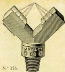
Головки газовых горелок Stadelmann из стеатитовой керамики (1906 г., Catalogue des becs Hella, музей Ultimheat)
